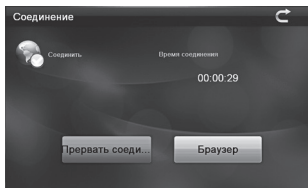
Рисунок 27. Интернет-соединение установлено
