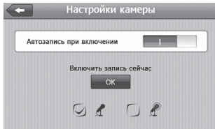
Рисунок 30. Настройки видеорегистратора
