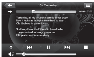
Рисунок 5. Интерфейс аудиопроигрывателя
