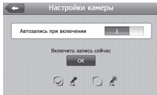
Рисунок 54. Настройки видеорегистратора
